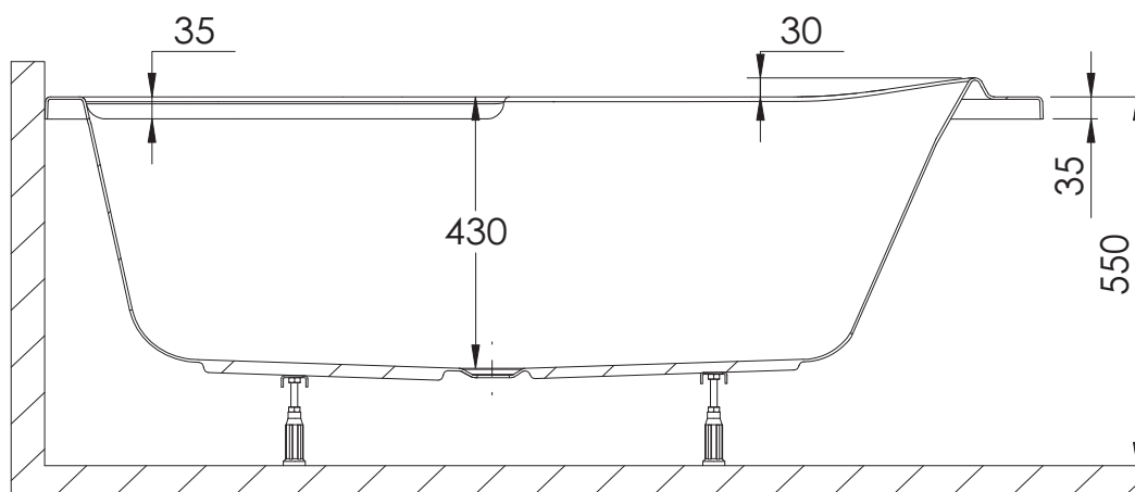
ŘEZ A-A
